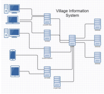
Gambar 4. Modul Sistem-informasi Desa
