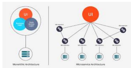
Gambar 1. Ilustrasi Perbedaan monolith dan microservices
