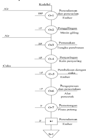
Gambar 3. Peta Proses Operasi Pembuatan Tahu UKM “SRT”
