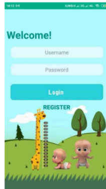
Gambar 3. Halaman Login
