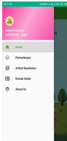
Gambar 4. Halaman Menu
