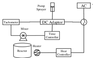
Gambar 4. Sistem elektrik reaktor
