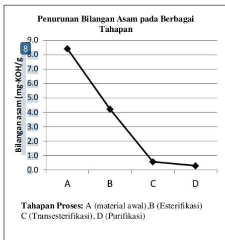
Gambar 9. Penurunan bilangan asam pada berbagai tahapan proses
