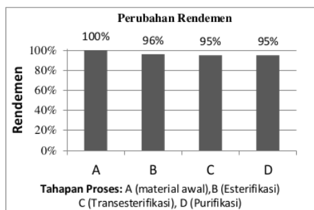
Gambar 10. Penurunan rendemen pada berbagai tahapan proses
