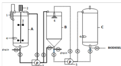
Gambar 3. Rangkaian reaktor biodiesel
