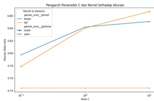
Gambar 4. Grafik pengaruh parameter C dan kernel terhadap akurasi
