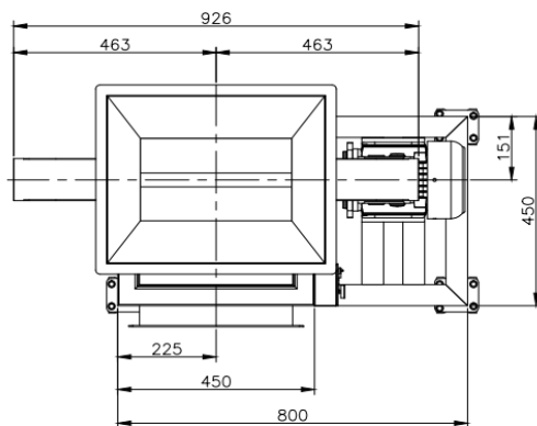
Desain Penampakan Dari Atas
