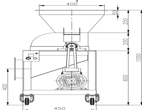
Desain Penampakan Dari Samping
