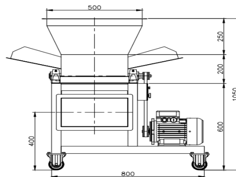
Desain Penampakan Dari Depan
