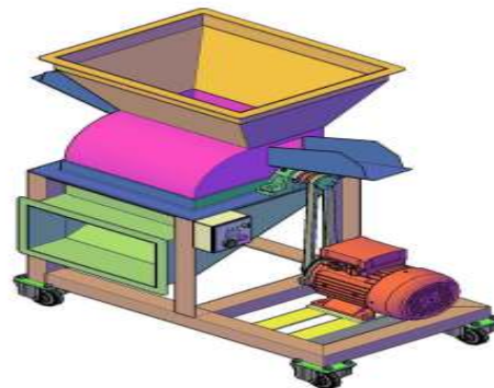
Desain Secara 3 Dimensi
