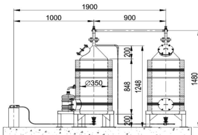
Gambar 5. Desain Pirolisis Konsep B Tampak Samping.
