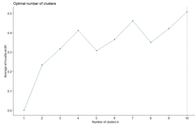
Gambar 2. Grafik Silhouette Coefficient dengan Jumlah Cluster 1 sampai 10
