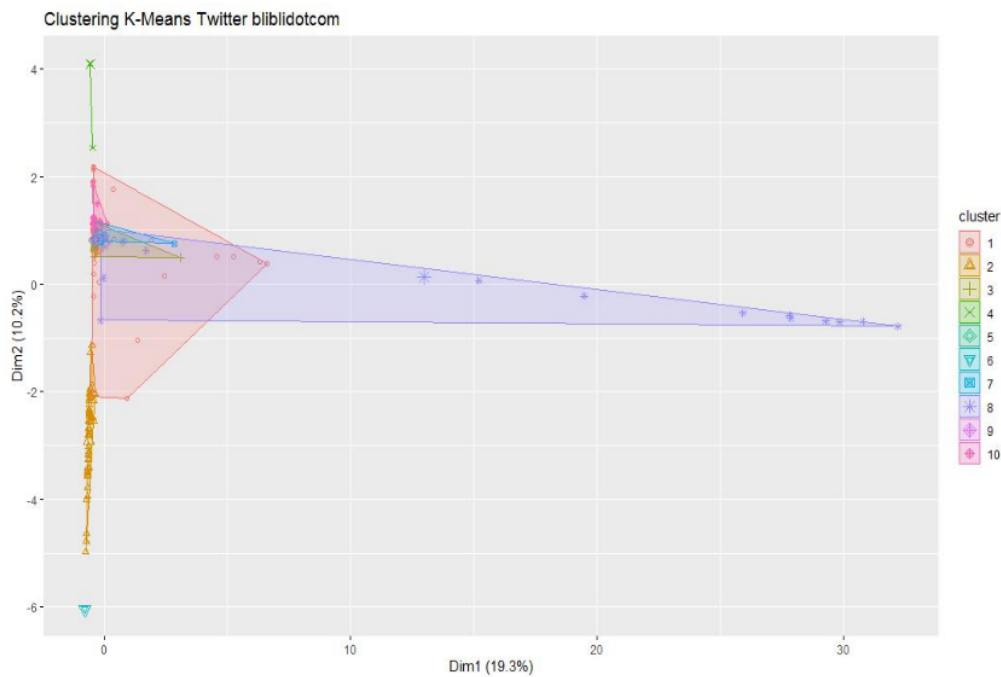
Gambar 3. Grafik Penyebaran Tweet blibliidotcom dalam 10 Cluster
