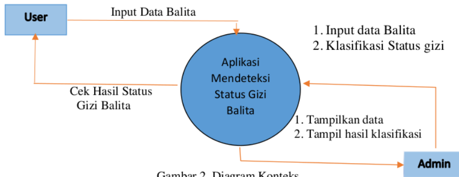
Gambar 2. Diagram Konteks
